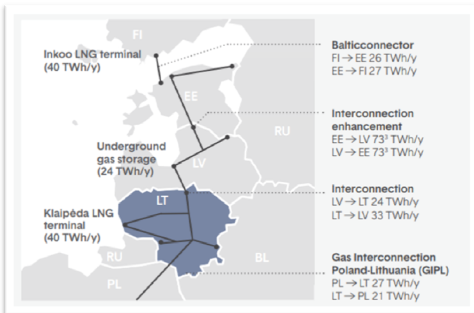
Рис. 10. Газовая инфраструктура в регионе
